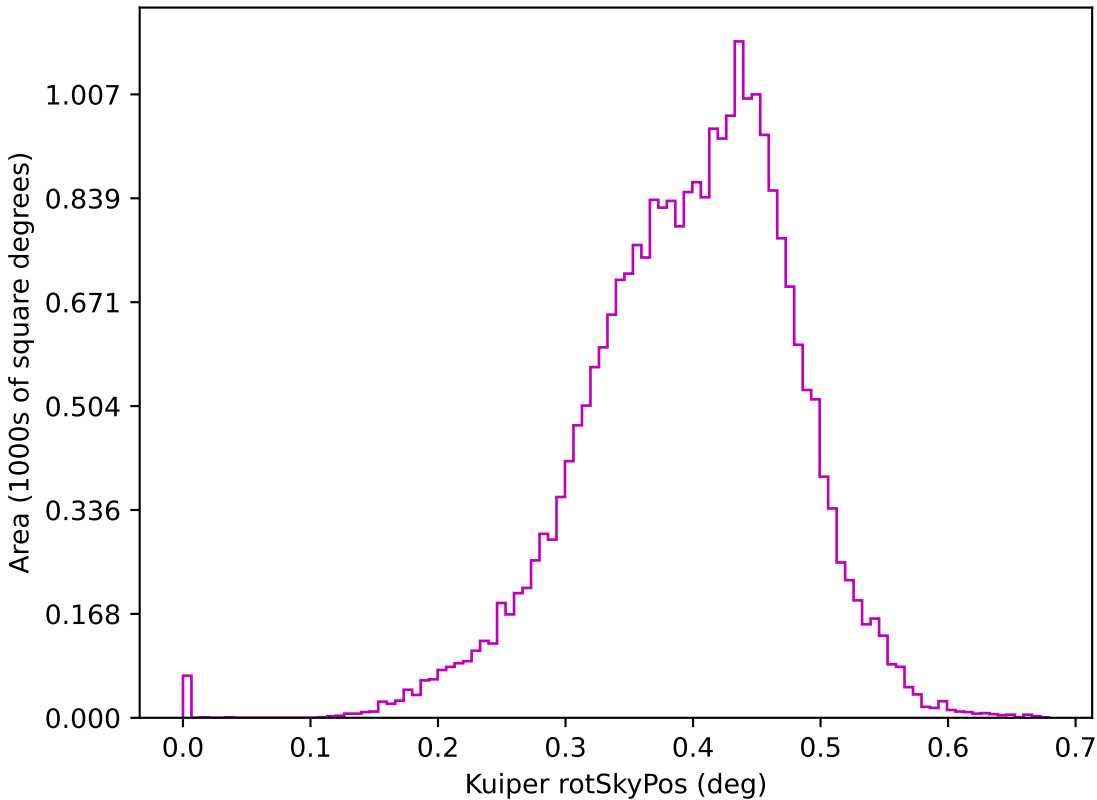
too_elab_r16_d3_ugrizy_v3.4_10yrs z: Kuiper rotSkyPos
