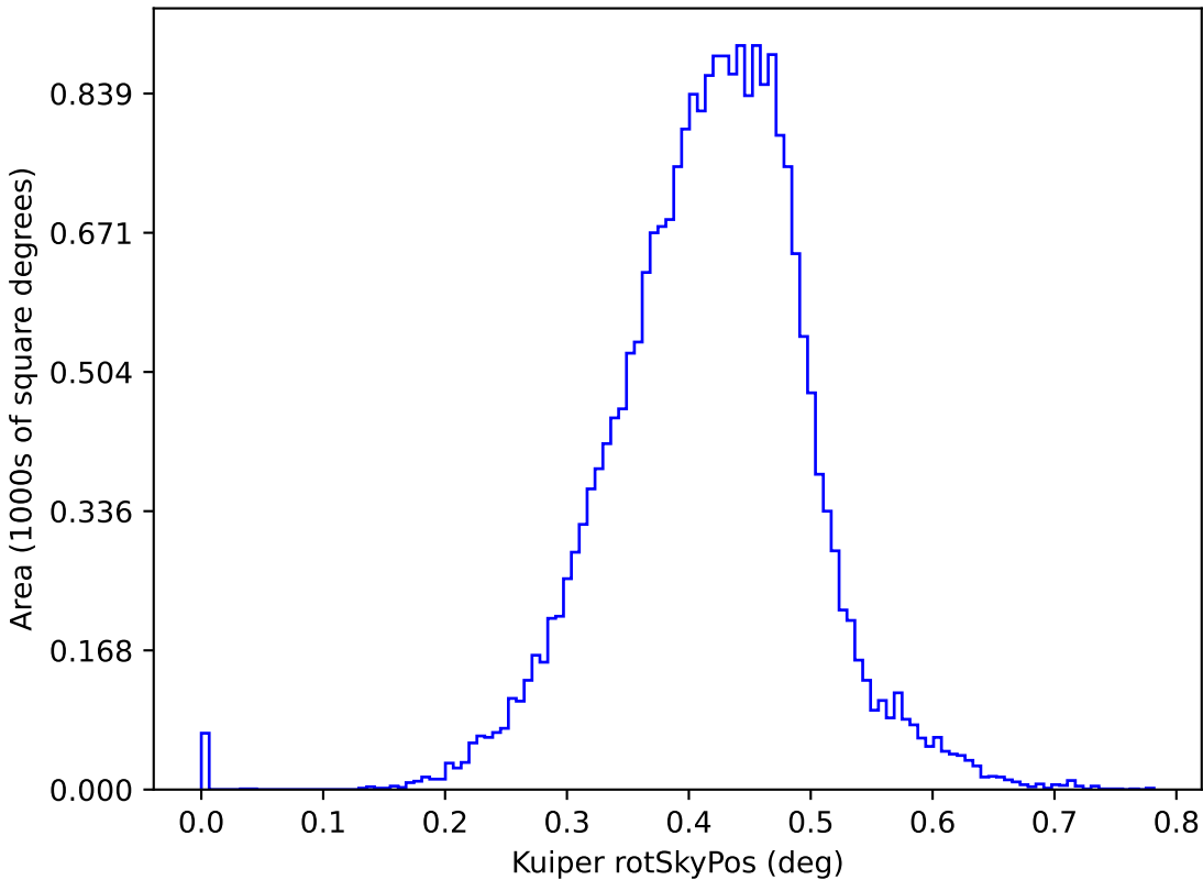
too_elab_r16_d3_ugrizy_v3.4_10yrs y: Kuiper rotSkyPos
