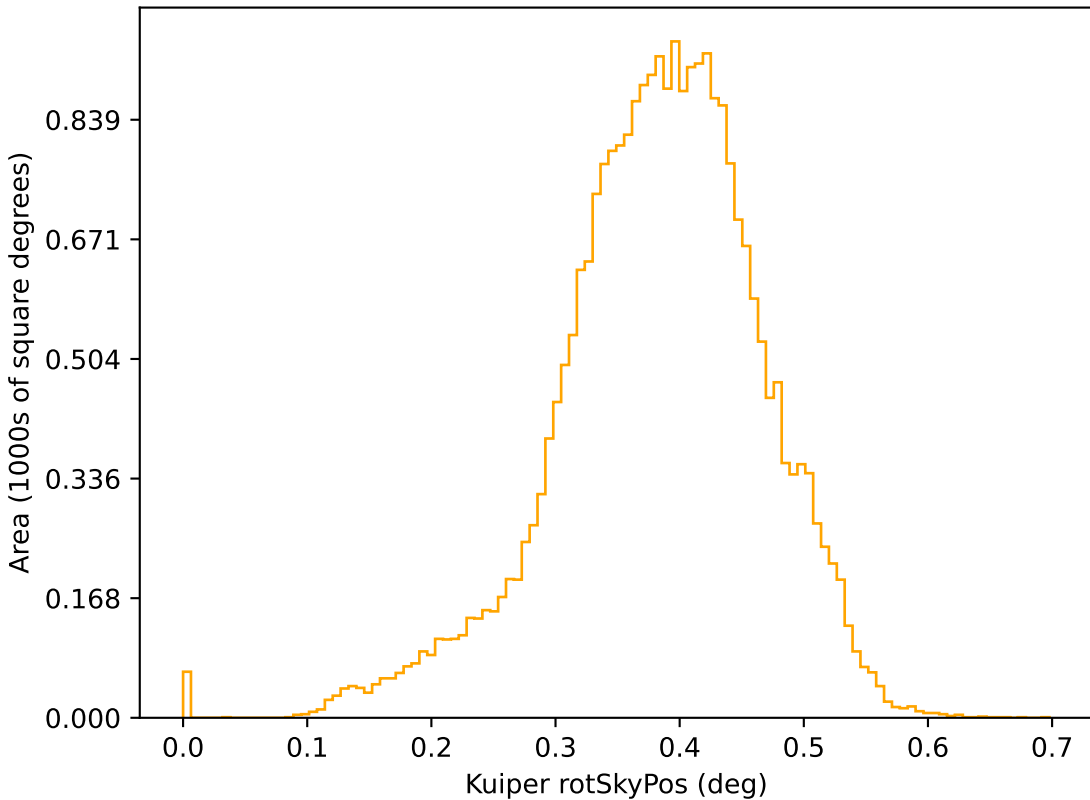
too_elab_r16_d3_ugrizy_v3.4_10yrs r: Kuiper rotSkyPos
