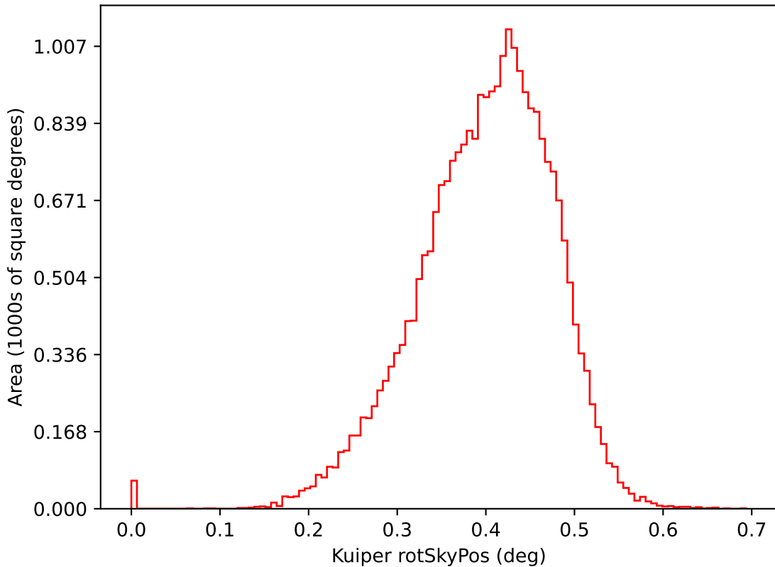
too_elab_r16_d3_ugrizy_v3.4_10yrs i: Kuiper rotSkyPos
