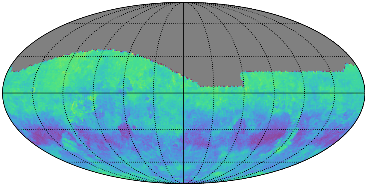
too_elab_r16_d3_ugrizy_v3.4_10yrs g: Kuiper rotSkyPos
