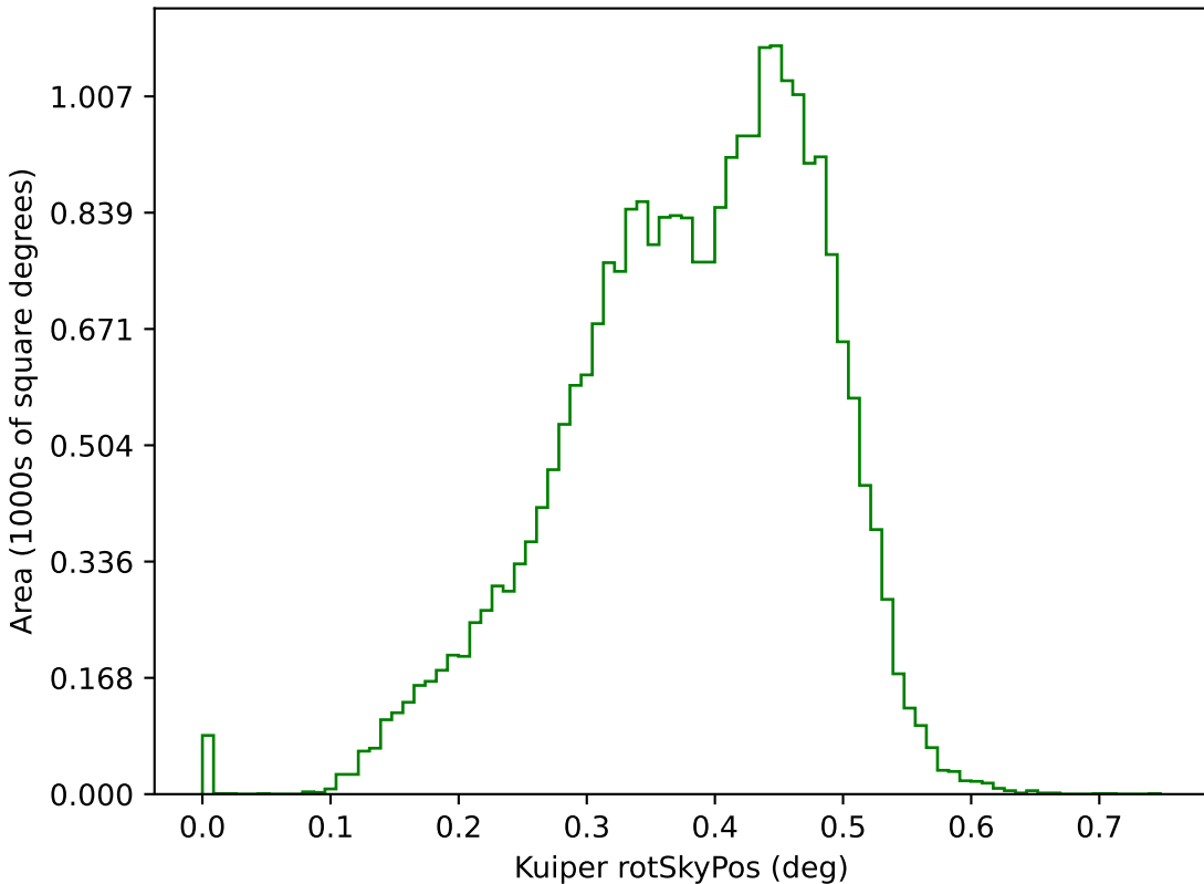
too_elab_r16_d3_ugrizy_v3.4_10yrs g: Kuiper rotSkyPos
