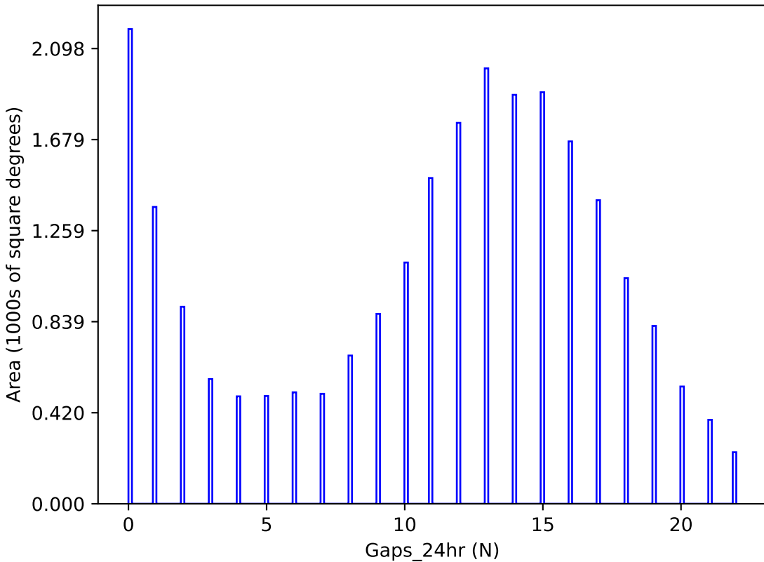
too_elab_r16_d3_ugrizy_v3.4_10yrs y band: Gaps_24hr
