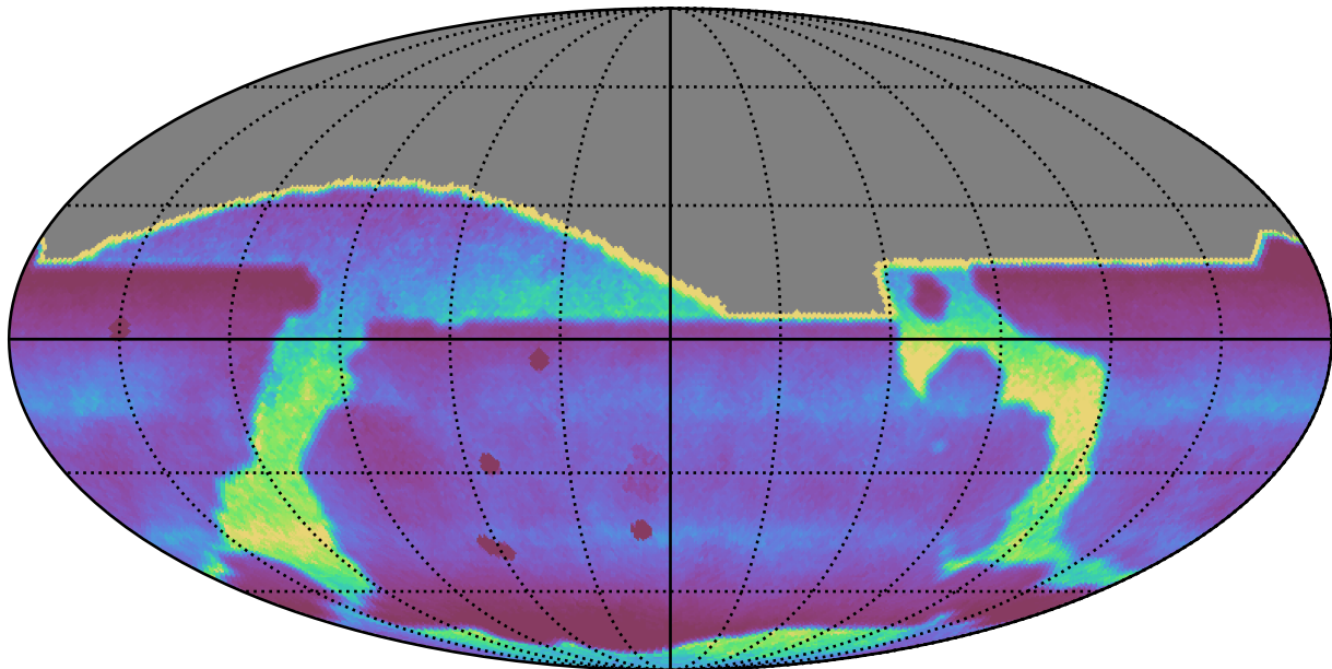
too_elab_r16_d3_ugrizy_v3.4_10yrs : DCRprecision
