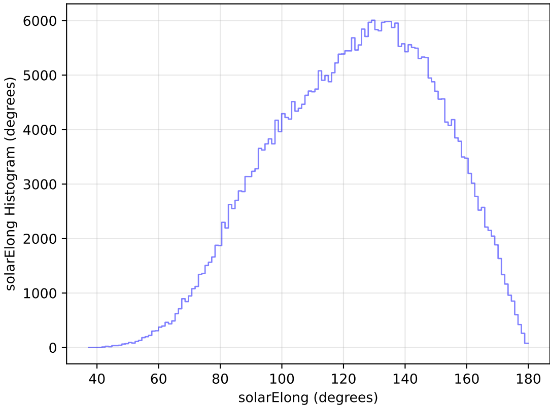
too_elab_r16_d3_ugrizy_v3.4_10yrs WFD y band: solarElong Histogram
