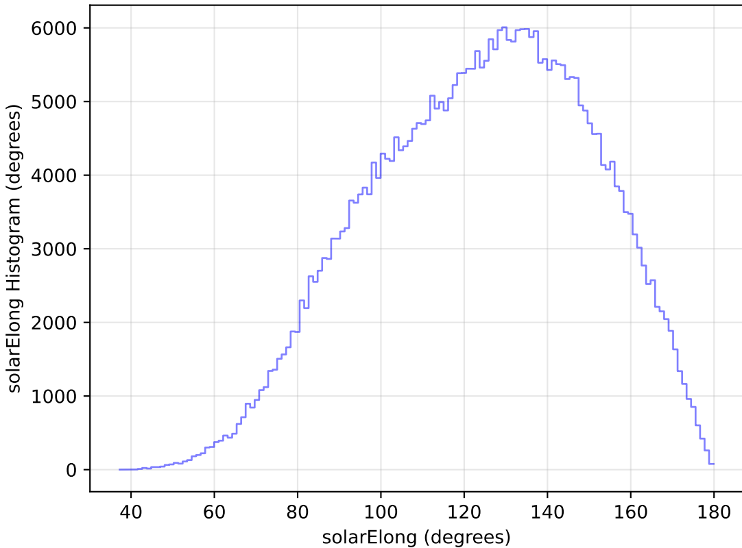
too_elab_r16_d3_ugrizy_v3.4_10yrs All sky y band: solarElong Histogram
