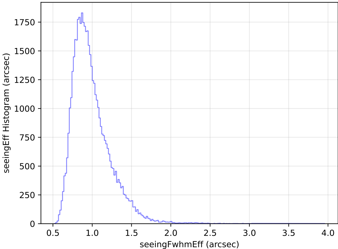
too_elab_r16_d3_ugrizy_v3.4_10yrs Yr 1 y band: seeingEff Histogram
