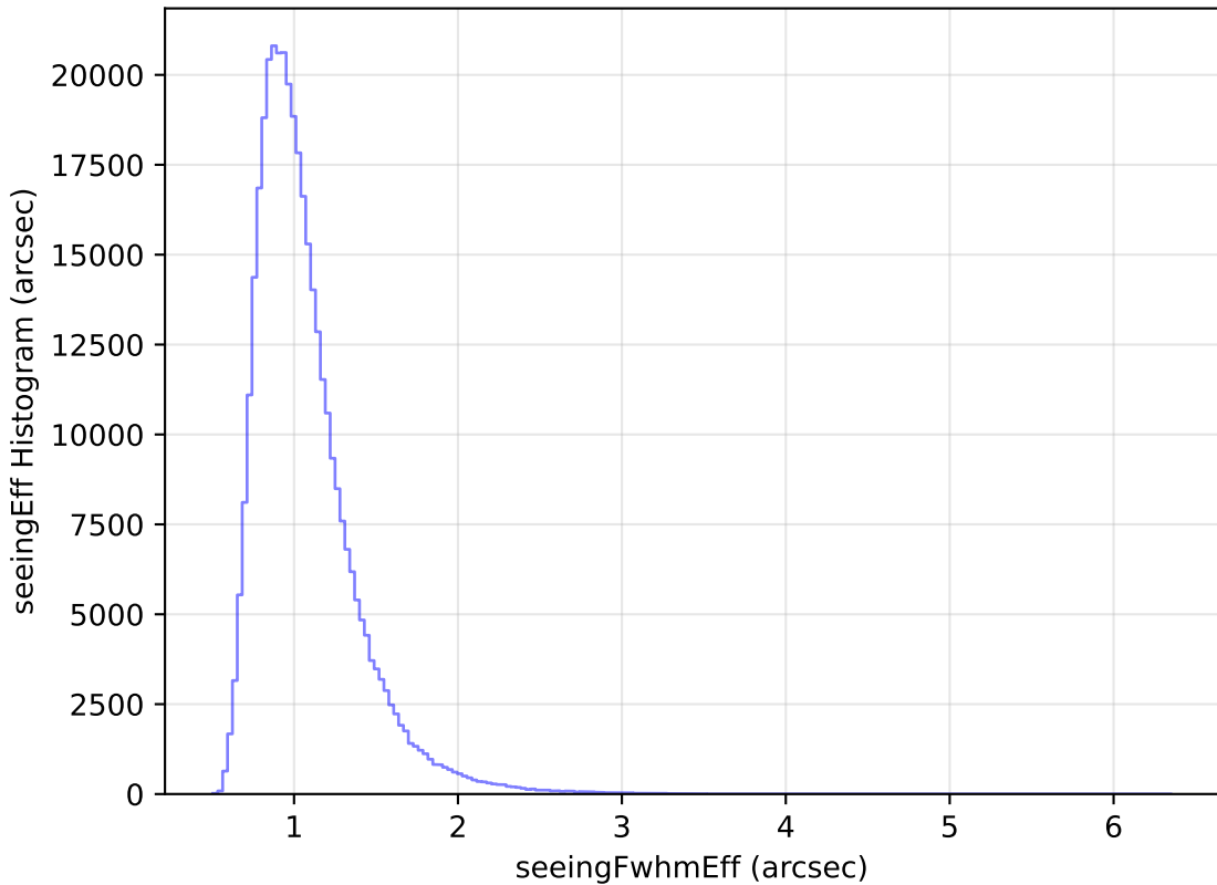
too_elab_r16_d3_ugrizy_v3.4_10yrs WFD y band: seeingEff Histogram
