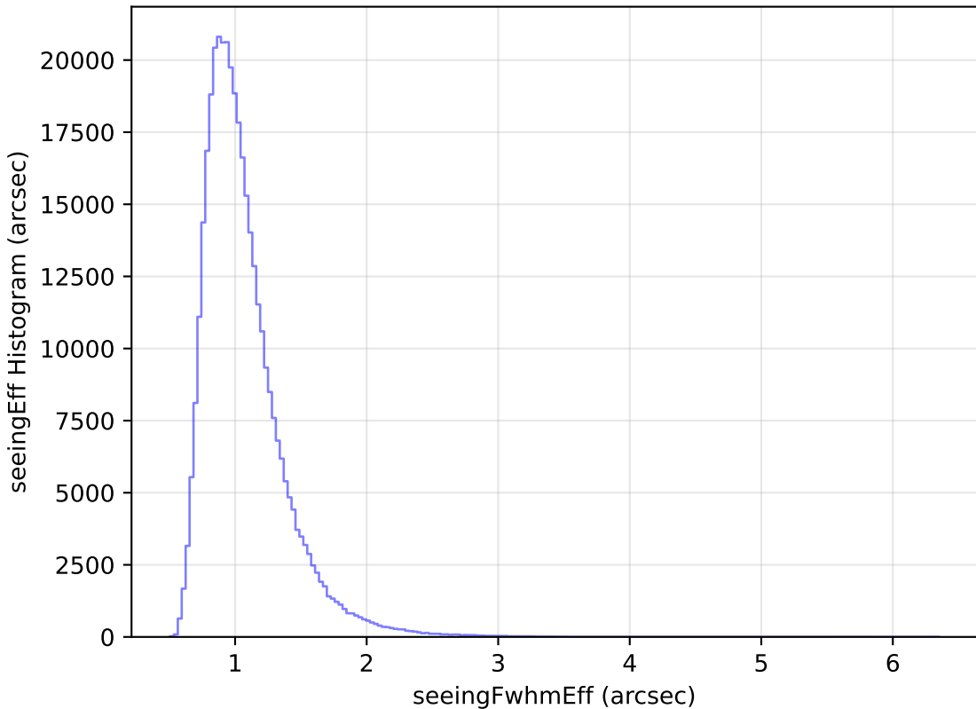
too_elab_r16_d3_ugrizy_v3.4_10yrs All sky y band: seeingEff Histogram
