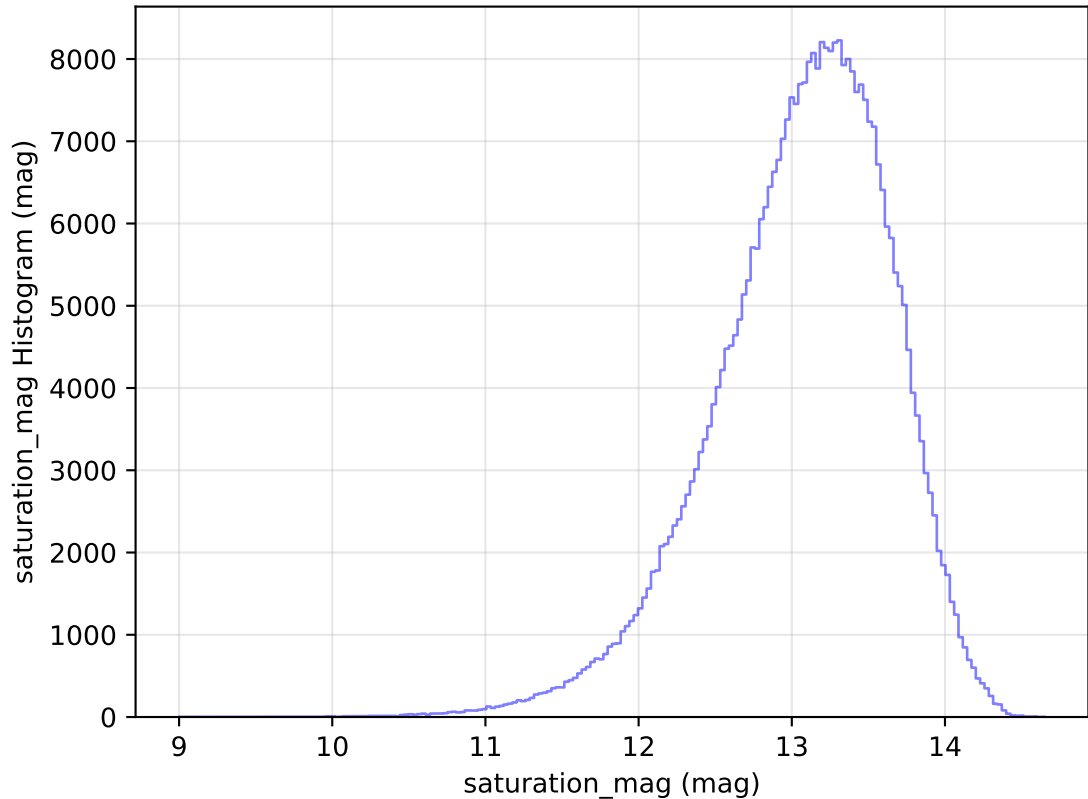
too_elab_r16_d3_ugrizy_v3.4_10yrs WFD y band: saturation_mag Histogram
