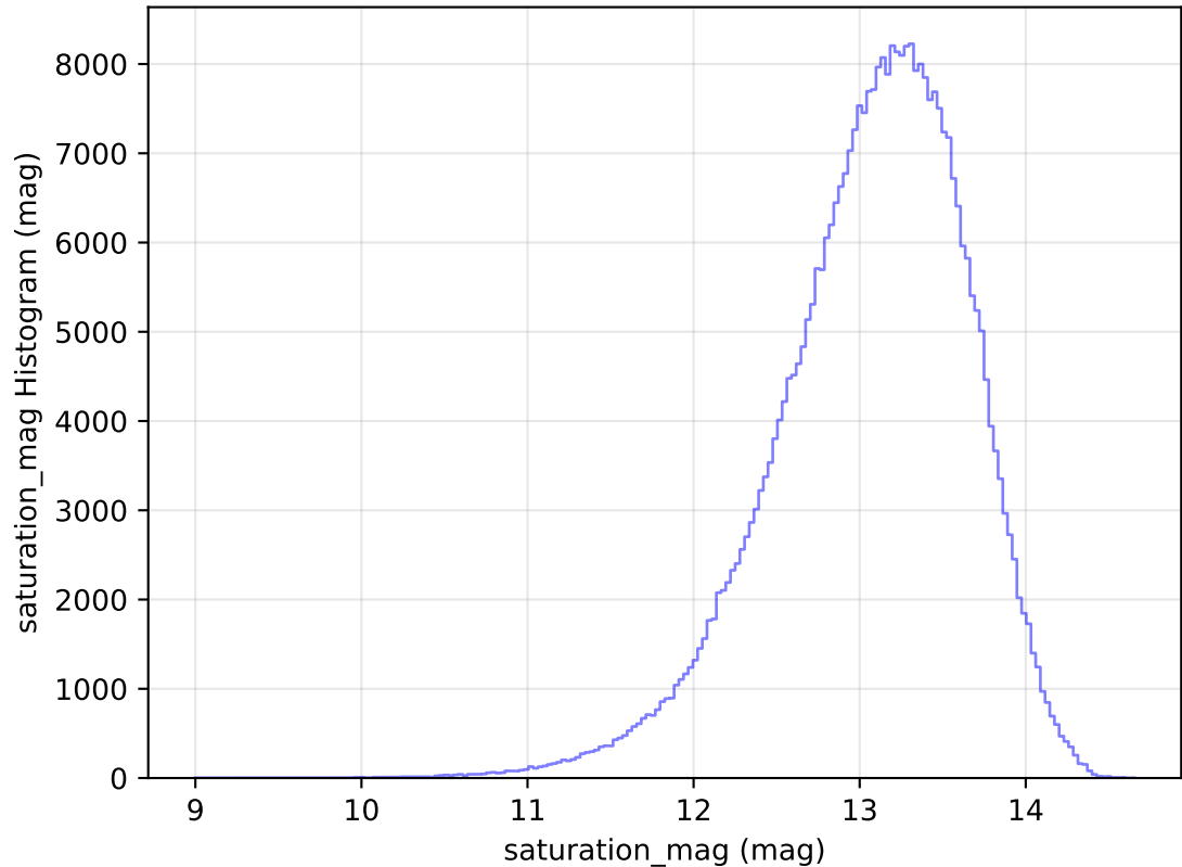
too_elab_r16_d3_ugrizy_v3.4_10yrs All sky y band: saturation_mag Histogram
