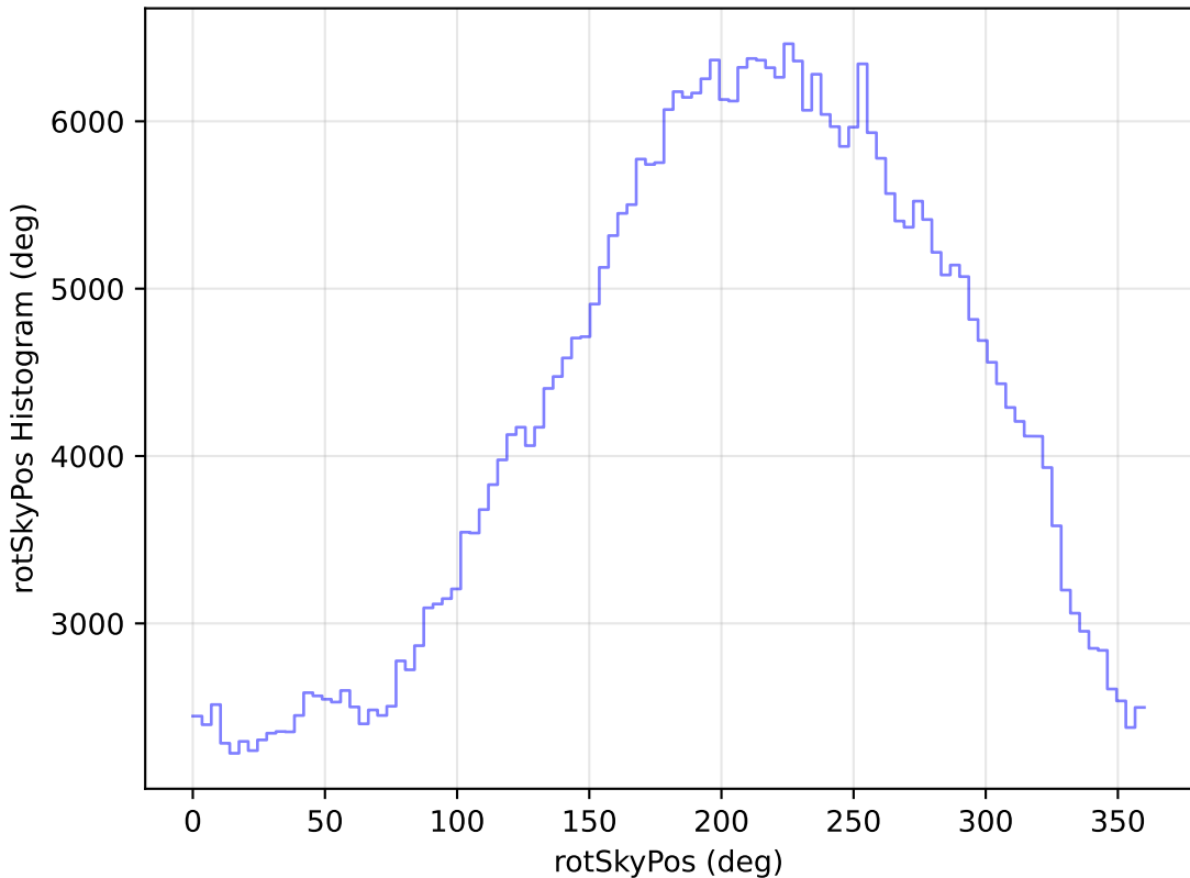
too_elab_r16_d3_ugrizy_v3.4_10yrs WFD z band: rotSkyPos Histogram
