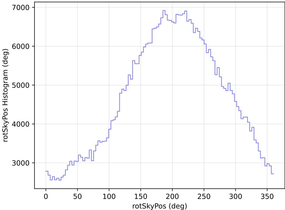
too_elab_r16_d3_ugrizy_v3.4_10yrs WFD r band: rotSkyPos Histogram
