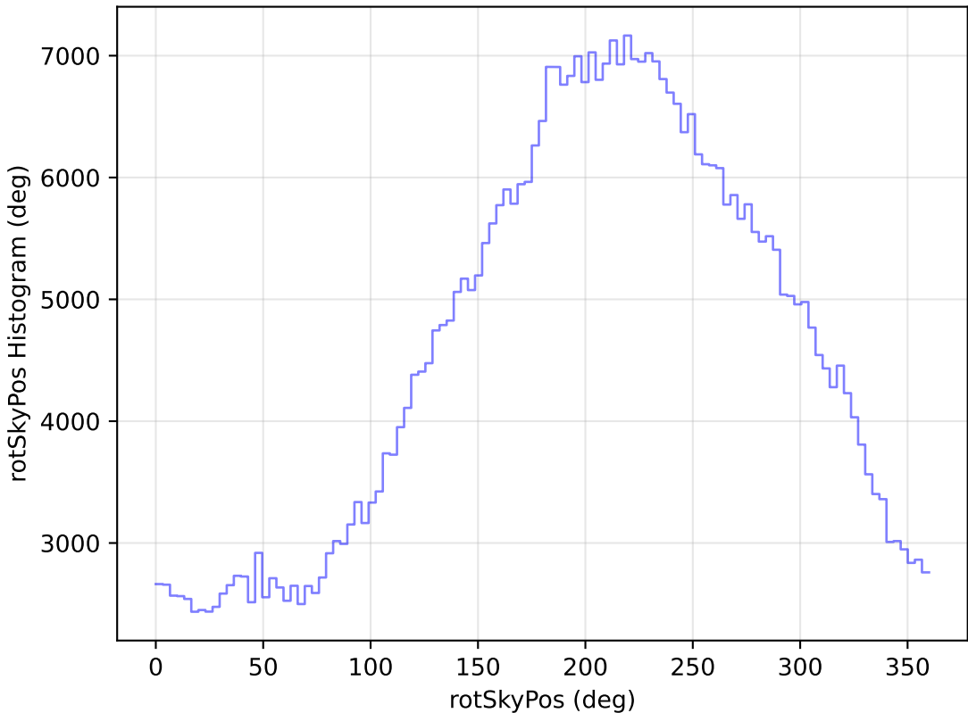
too_elab_r16_d3_ugrizy_v3.4_10yrs WFD i band: rotSkyPos Histogram
