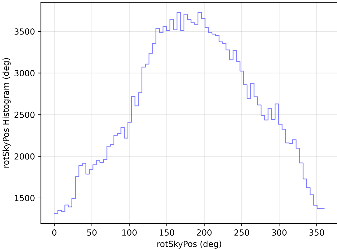
too_elab_r16_d3_ugrizy_v3.4_10yrs WFD g band: rotSkyPos Histogram
