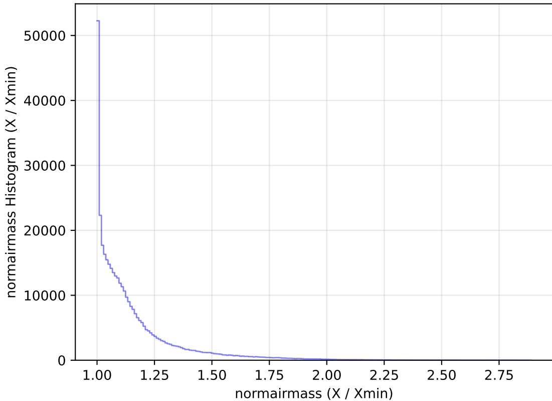
too_elab_r16_d3_ugrizy_v3.4_10yrs WFD y band: normairmass Histogram
