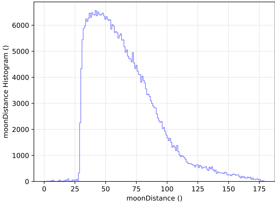
too_elab_r16_d3_ugrizy_v3.4_10yrs All sky y band: moonDistance Histogram
