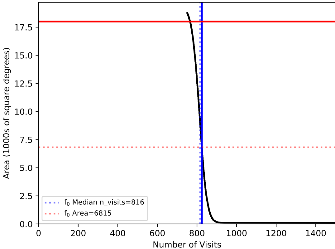
too_elab_r16_d3_ugrizy_v3.4_10yrs WFD: f0
