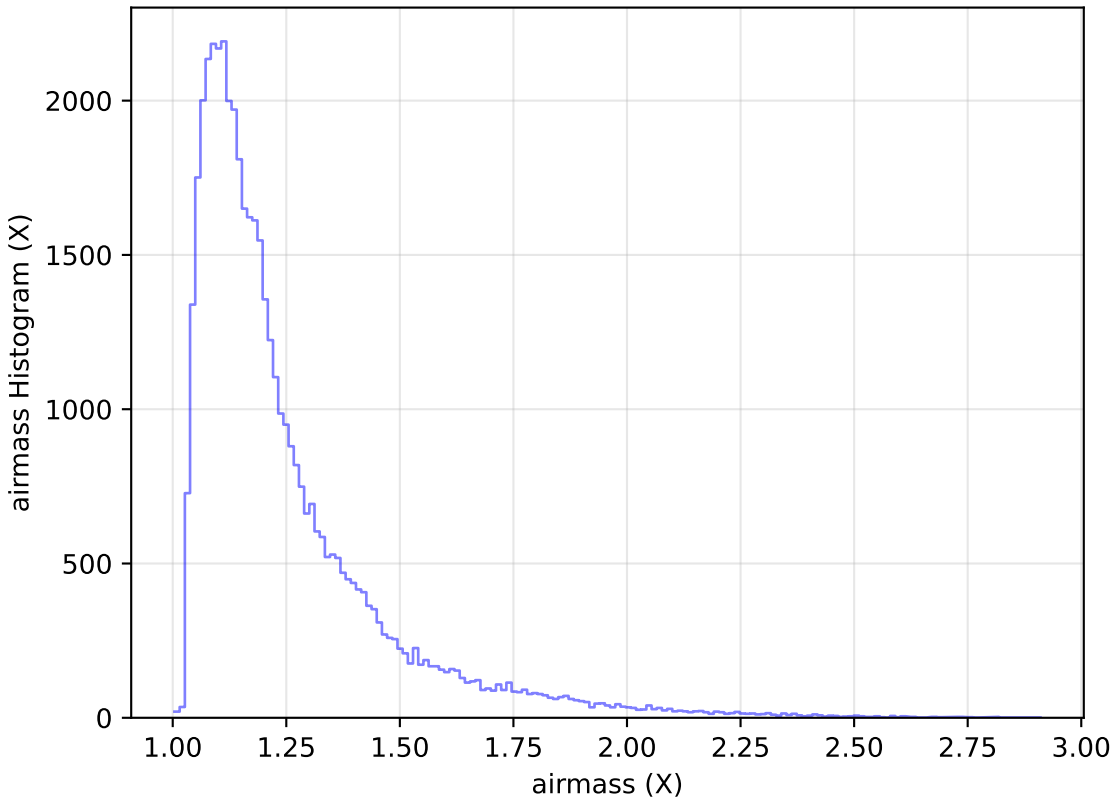
too_elab_r16_d3_ugrizy_v3.4_10yrs Yr 1 y band: airmass Histogram
