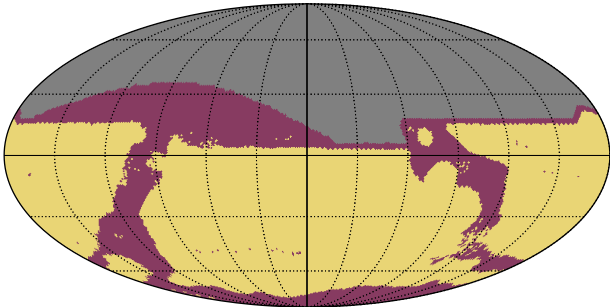
too_elab_r16_d3_ugrizy_v3.4_10yrs All sky: RapidRevisits
