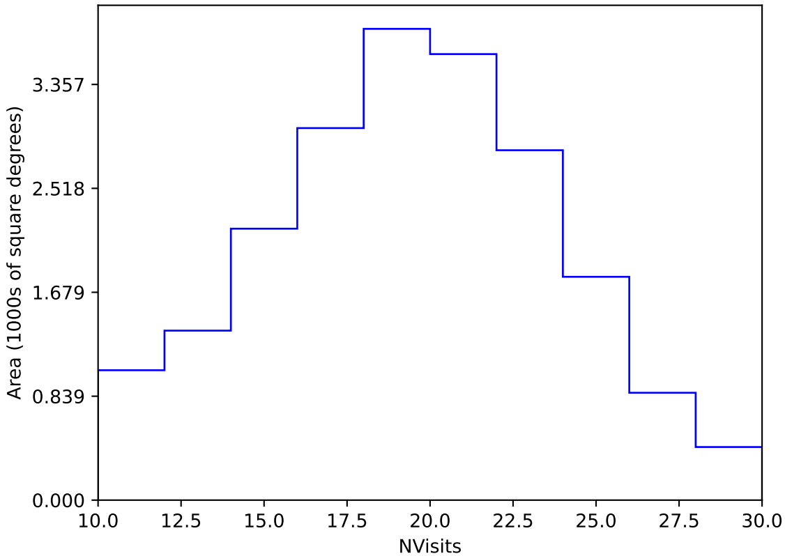
too_elab_r16_d3_ugrizy_v3.4_10yrs Yr 1 y band: NVisits
