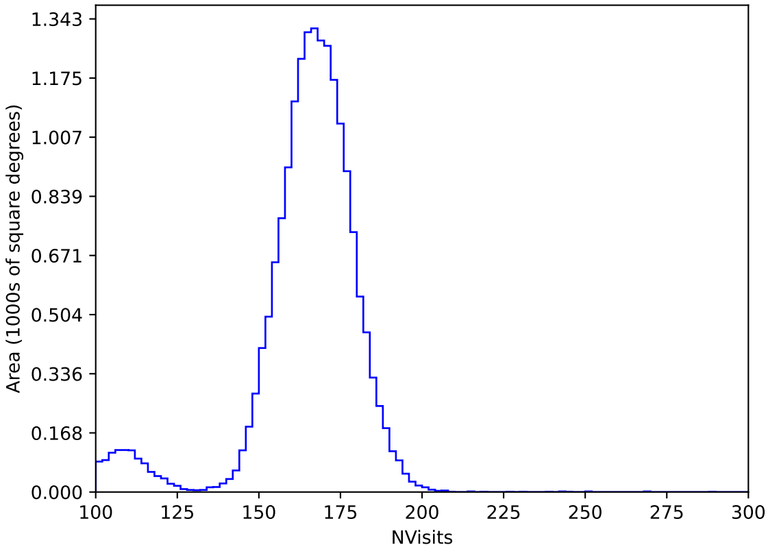
too_elab_r16_d3_ugrizy_v3.4_10yrs WFD y band: NVisits
