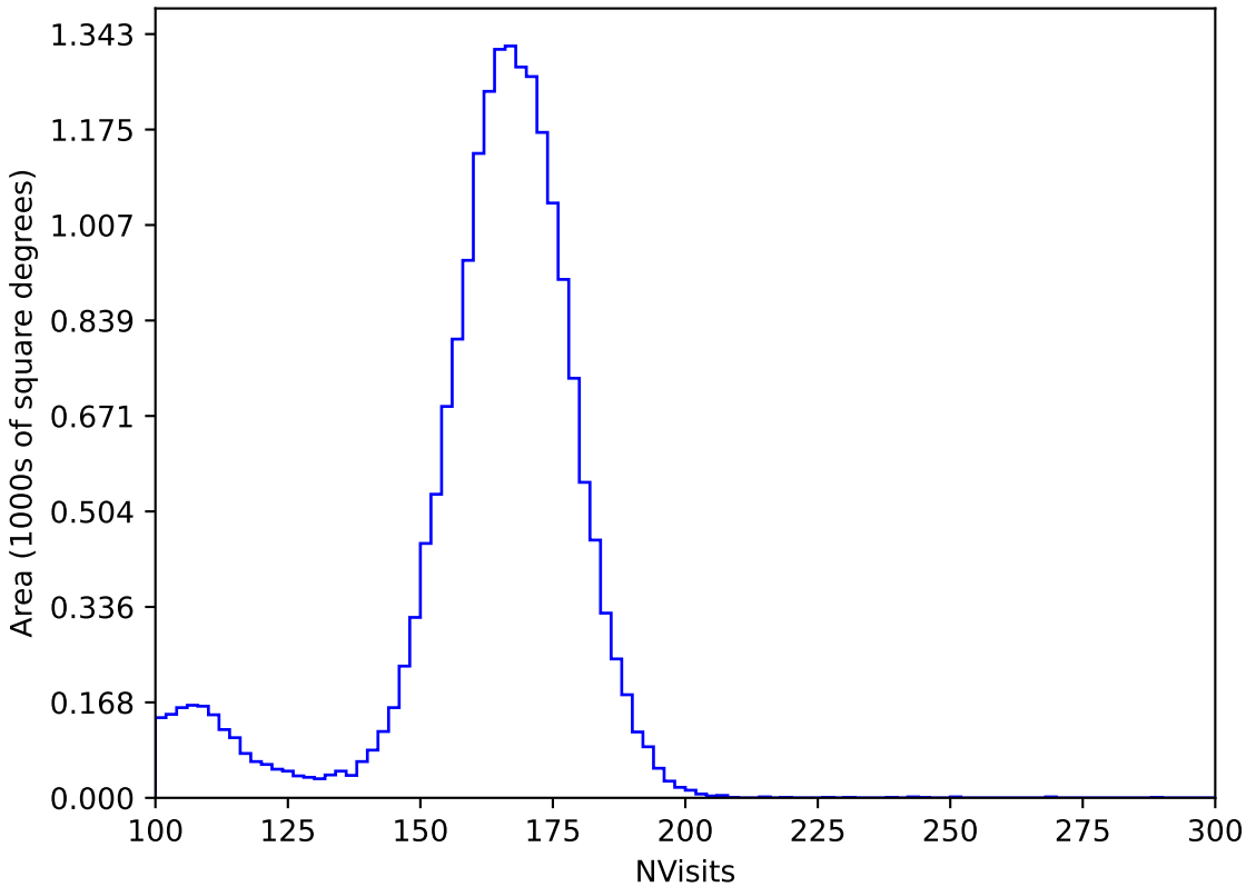
too_elab_r16_d3_ugrizy_v3.4_10yrs All sky y band: NVisits
