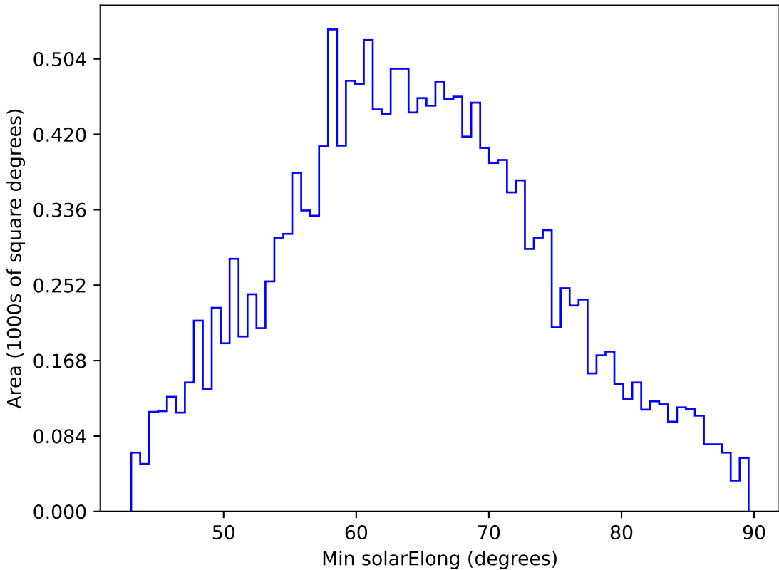
too_elab_r16_d3_ugrizy_v3.4_10yrs WFD y band: Min solarElong
