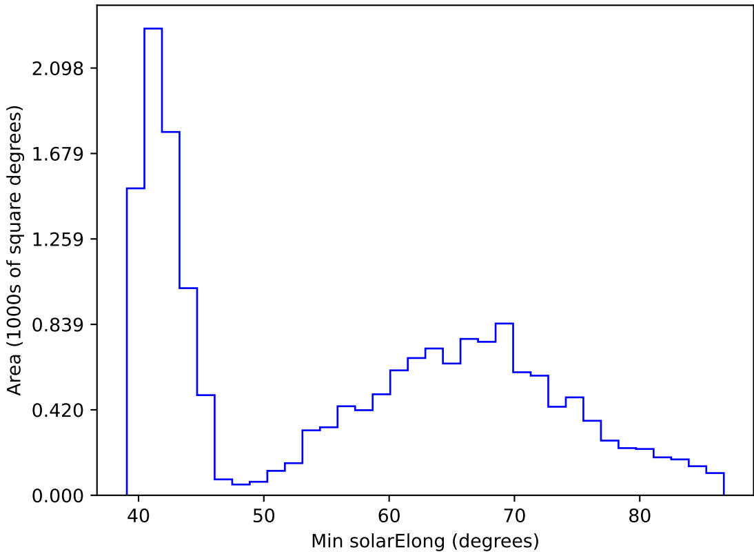
too_elab_r16_d3_ugrizy_v3.4_10yrs WFD r band: Min solarElong
