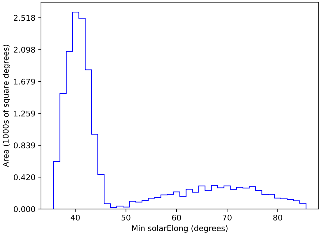
too_elab_r16_d3_ugrizy_v3.4_10yrs WFD i band: Min solarElong
