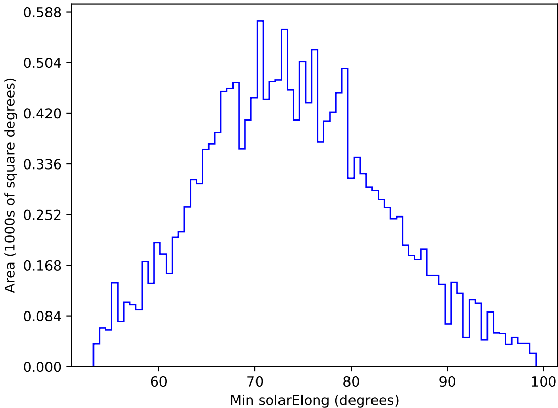
too_elab_r16_d3_ugrizy_v3.4_10yrs WFD g band: Min solarElong
