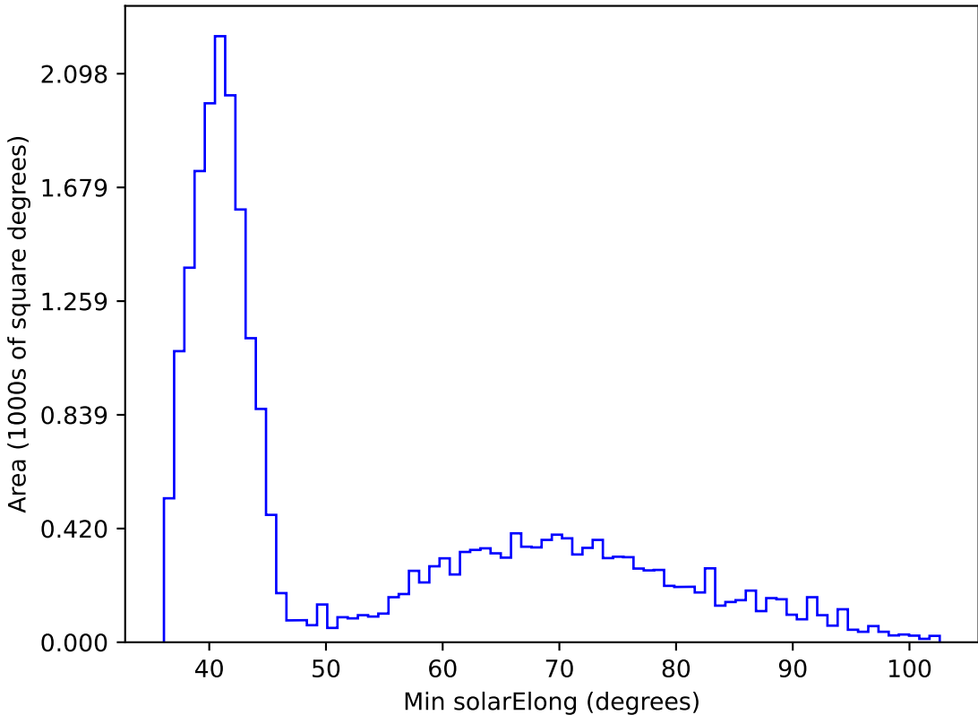
too_elab_r16_d3_ugrizy_v3.4_10yrs All sky z band: Min solarElong
