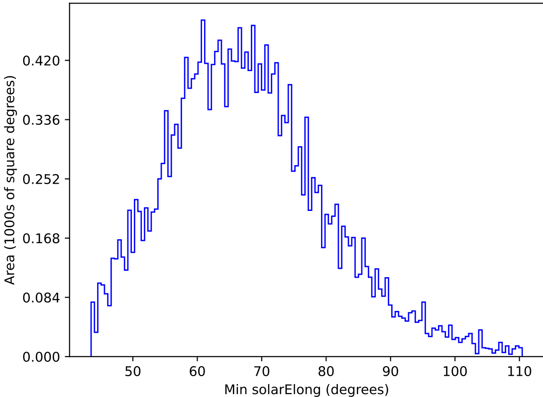
too_elab_r16_d3_ugrizy_v3.4_10yrs All sky y band: Min solarElong
