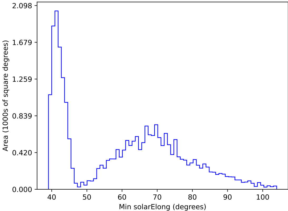
too_elab_r16_d3_ugrizy_v3.4_10yrs All sky r band: Min solarElong
