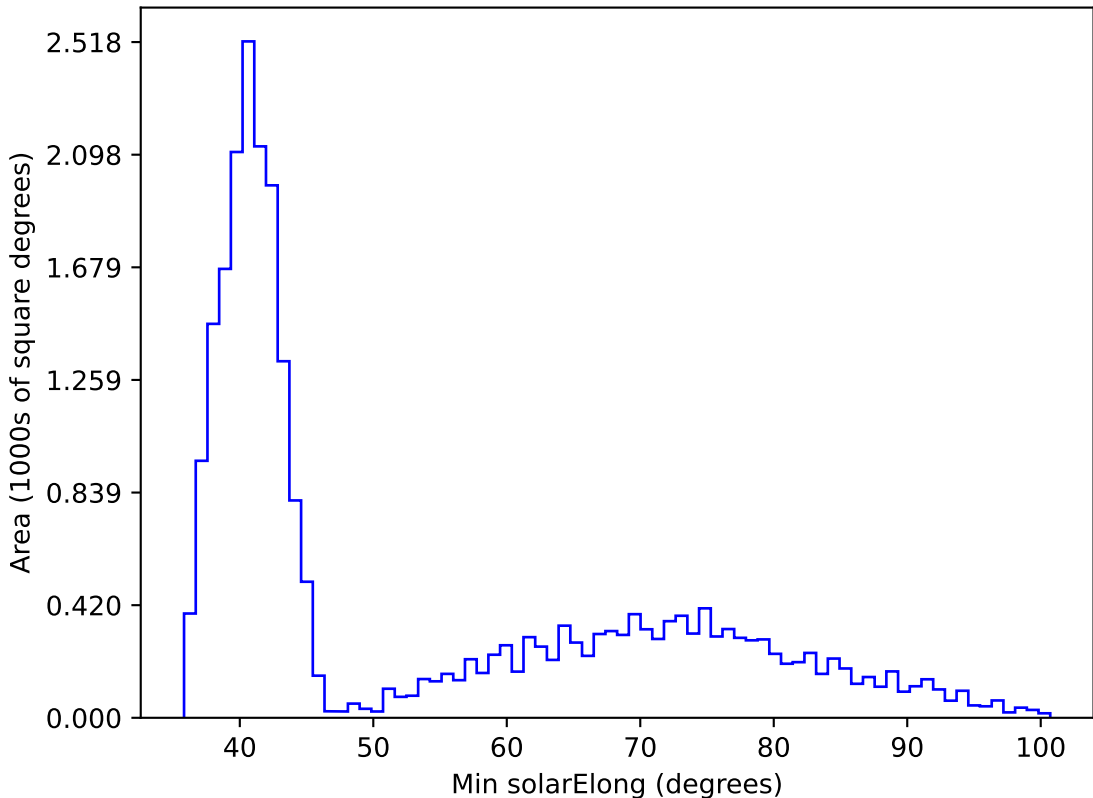
too_elab_r16_d3_ugrizy_v3.4_10yrs All sky i band: Min solarElong
