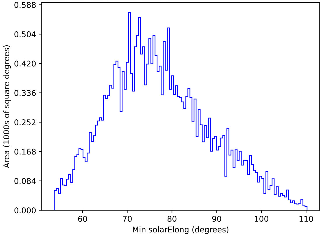
too_elab_r16_d3_ugrizy_v3.4_10yrs All sky g band: Min solarElong
