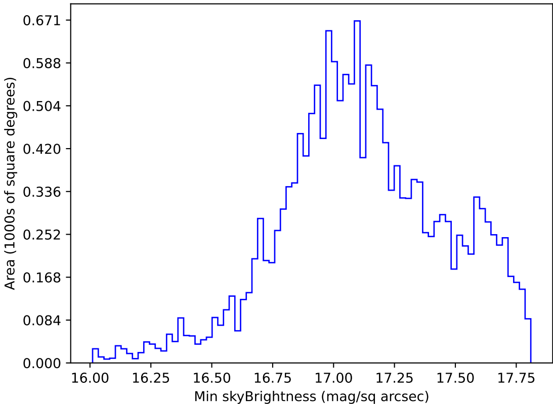
too_elab_r16_d3_ugrizy_v3.4_10yrs WFD y band: Min skyBrightness
