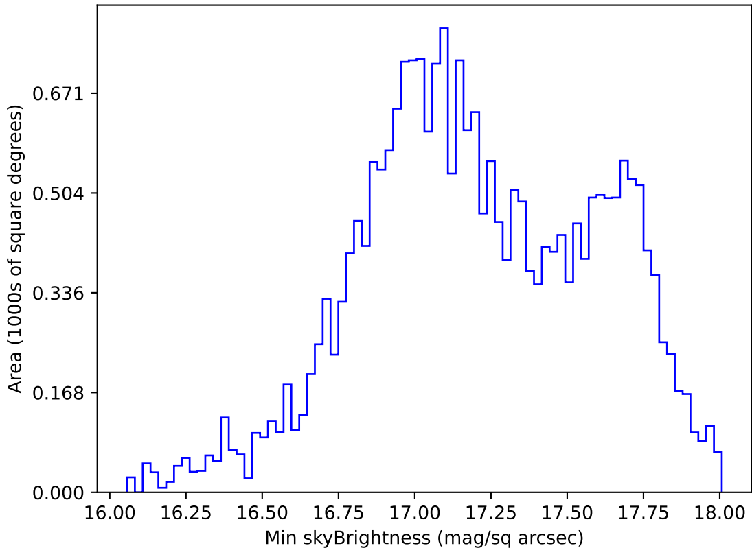
too_elab_r16_d3_ugrizy_v3.4_10yrs All sky y band: Min skyBrightness
