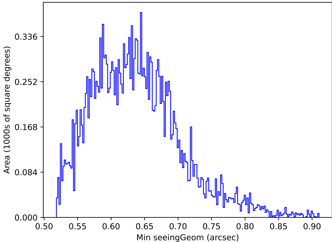
too_elab_r16_d3_ugrizy_v3.4_10yrs Yr 1 y band: Min seeingGeom
