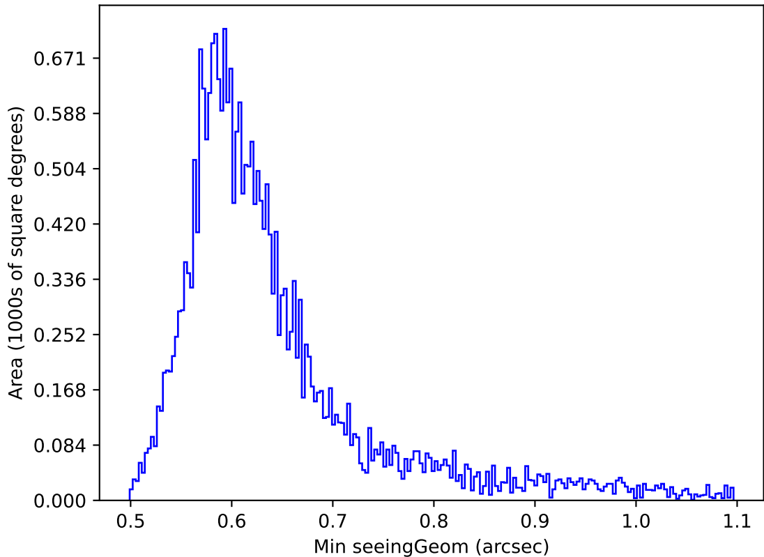
too_elab_r16_d3_ugrizy_v3.4_10yrs Yr 1 i band: Min seeingGeom
