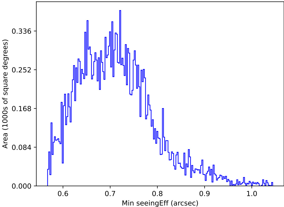
too_elab_r16_d3_ugrizy_v3.4_10yrs Yr 1 y band: Min seeingEff
