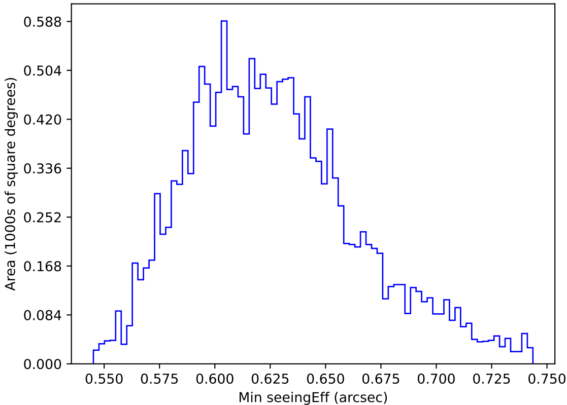
too_elab_r16_d3_ugrizy_v3.4_10yrs WFD y band: Min seeingEff
