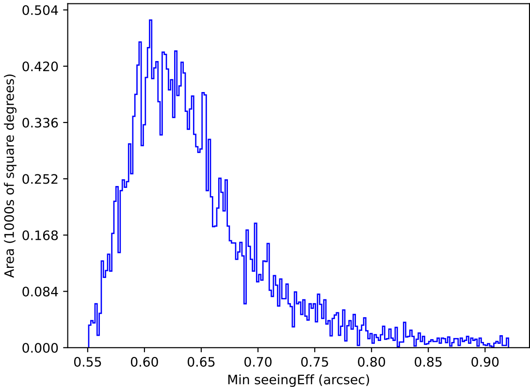
too_elab_r16_d3_ugrizy_v3.4_10yrs All sky y band: Min seeingEff
