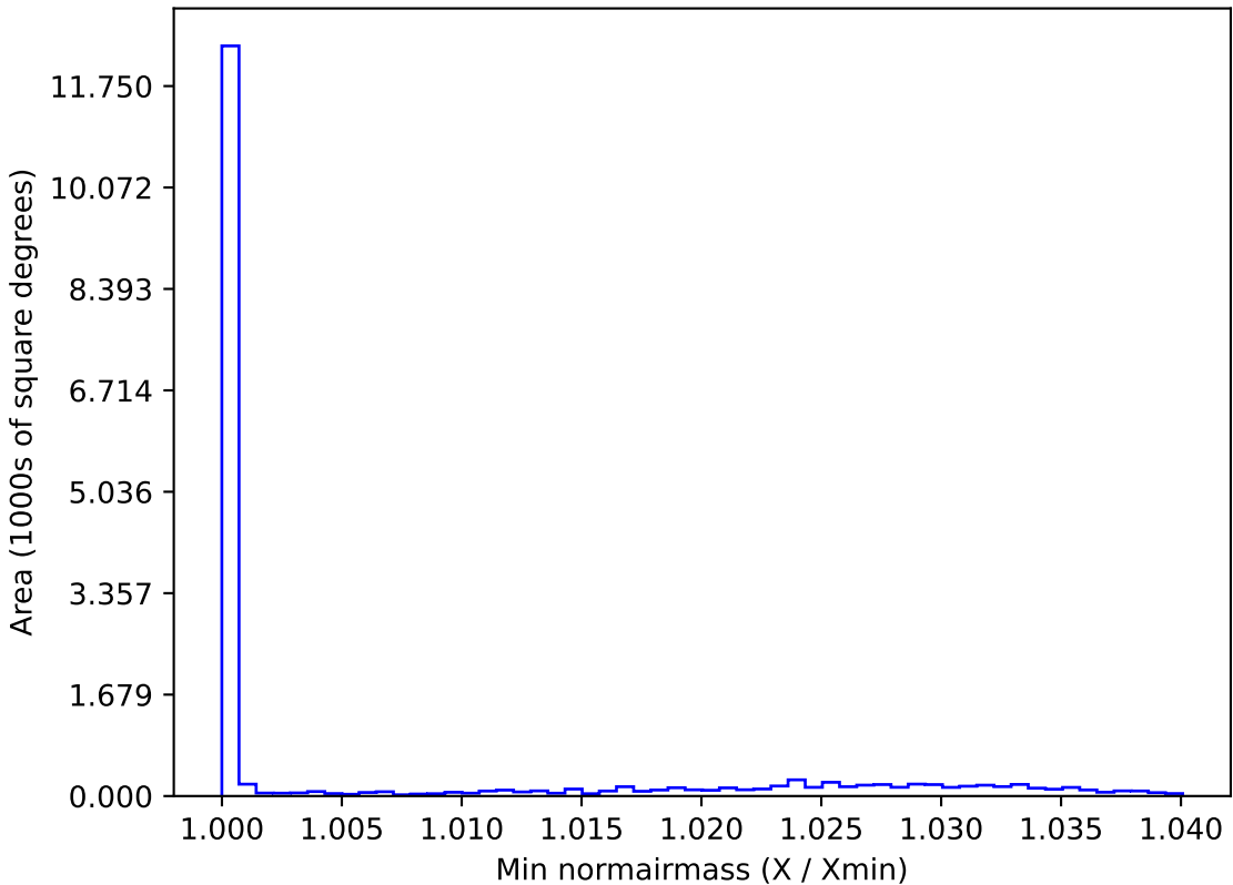
too_elab_r16_d3_ugrizy_v3.4_10yrs WFD y band: Min normairmass
