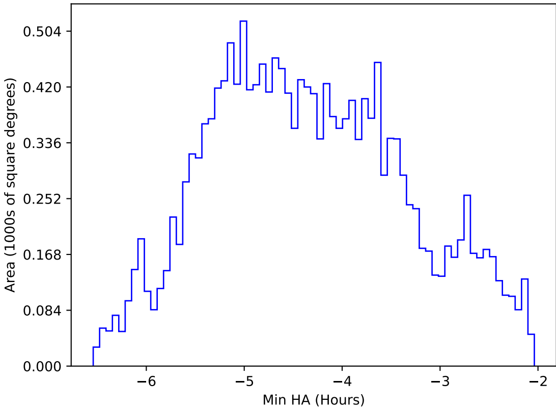
too_elab_r16_d3_ugrizy_v3.4_10yrs WFD z band: Min HA
