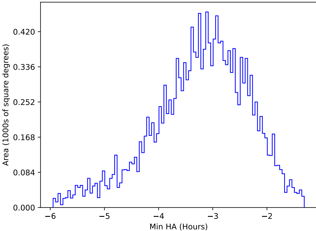
too_elab_r16_d3_ugrizy_v3.4_10yrs WFD u band: Min HA
