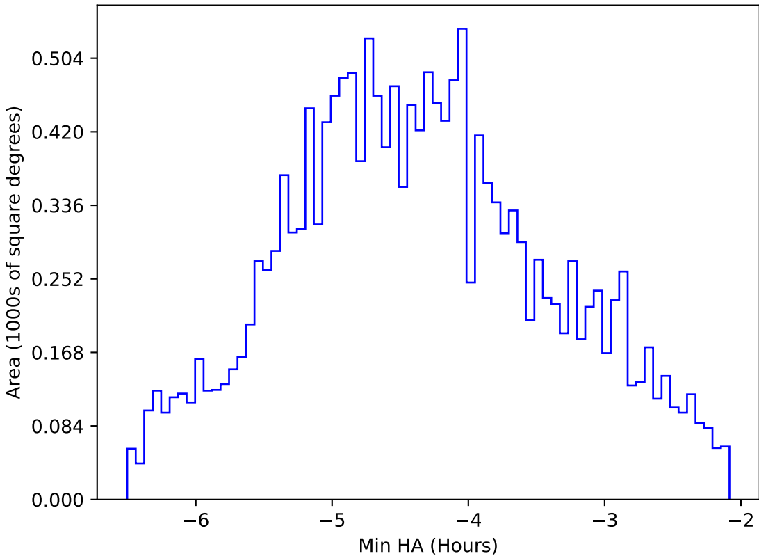
too_elab_r16_d3_ugrizy_v3.4_10yrs WFD i band: Min HA
