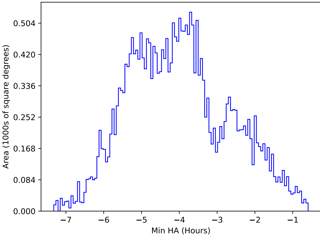
too_elab_r16_d3_ugrizy_v3.4_10yrs All sky z band: Min HA
