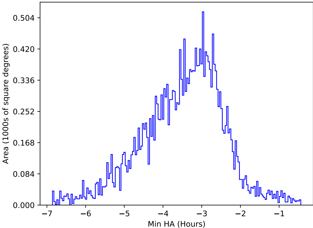
too_elab_r16_d3_ugrizy_v3.4_10yrs All sky y band: Min HA
