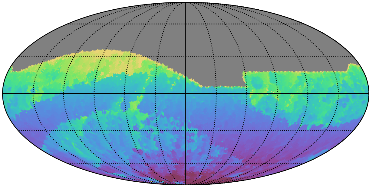
too_elab_r16_d3_ugrizy_v3.4_10yrs All sky r band: Min HA
